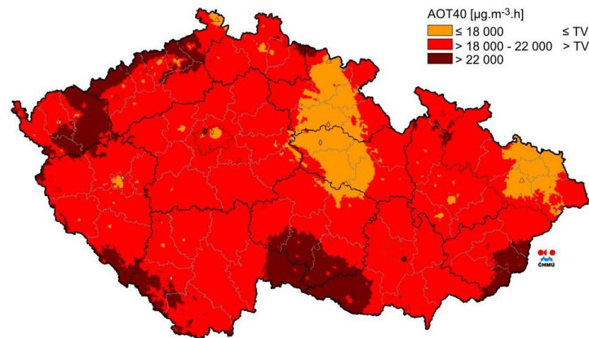
ozone: AOT40 2005-2008
