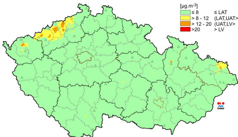
SO 2 2008
