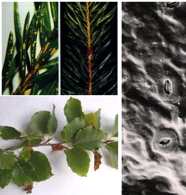
SO 2 2008
